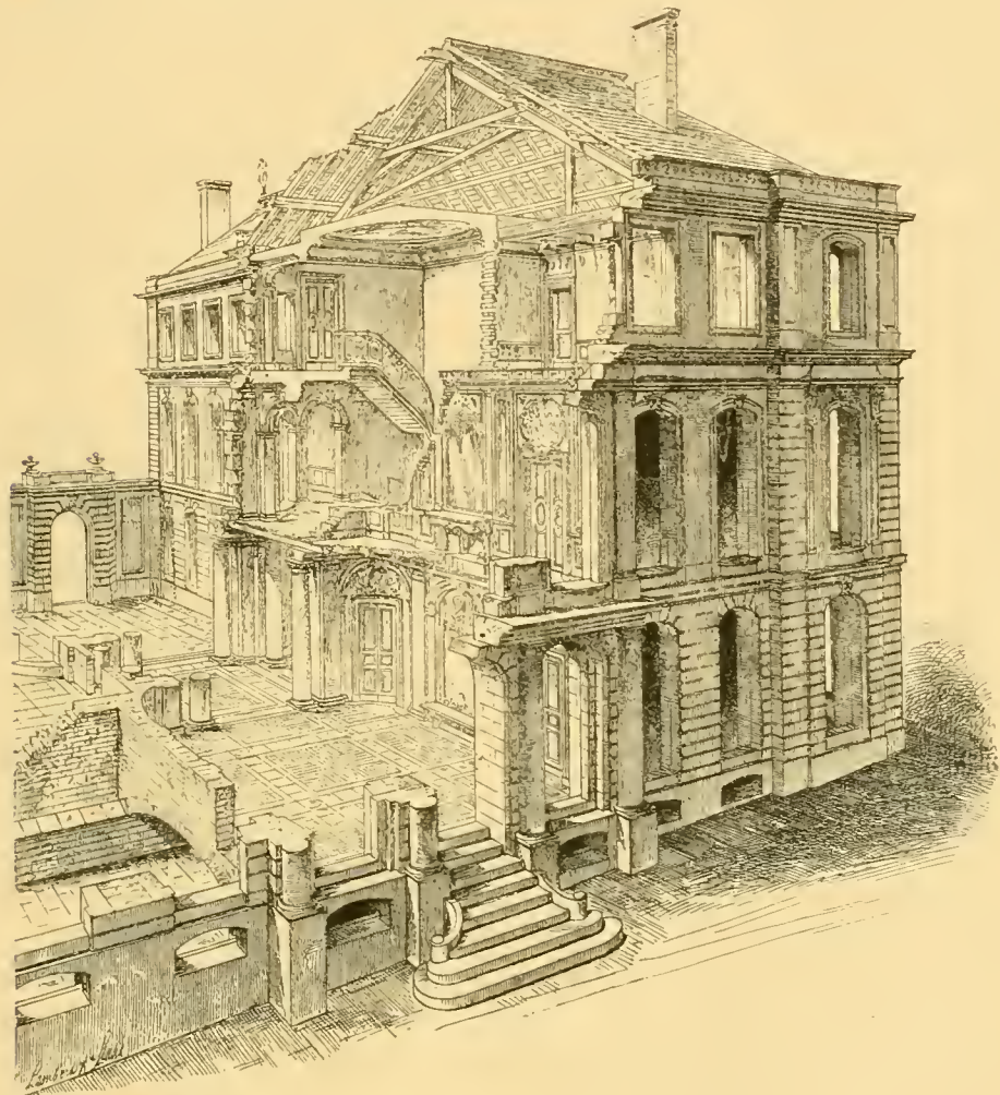
Fig. 161. Hôtel Mallet zu Genf. Perspektivischer Querschnitt.
